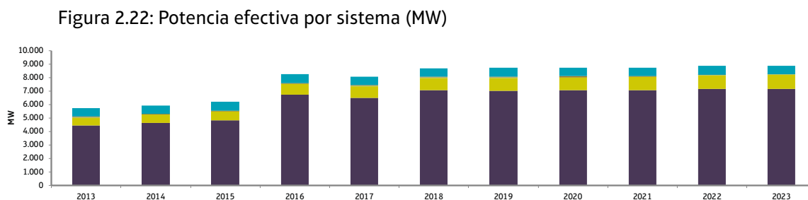
Figura 2.22: Potencia efectiva por sistema (MW)
