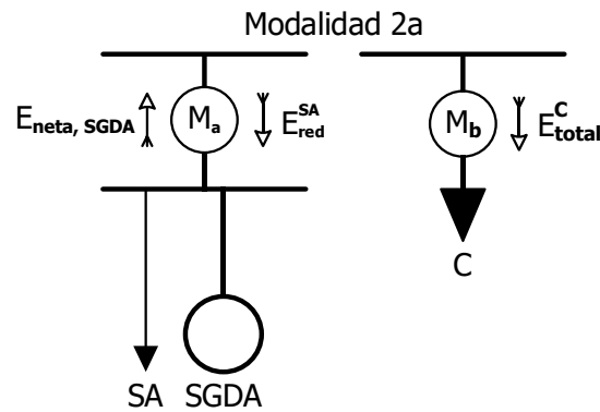
Ilustración 5. Diagrama de la Modalidad 2a (SGDA y consumidor regulado ubicados en inmuebles diferentes) con medidores M_a y M_b
